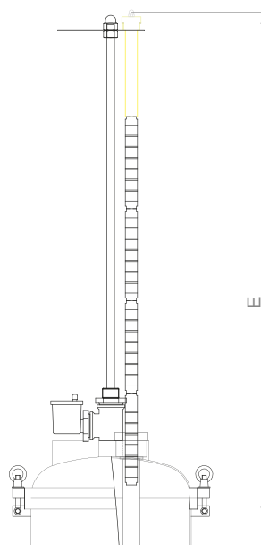
Testa rotante per lavaggio candele magnetiche e filtro meccanico
